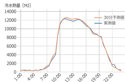
代表日の熱需要量グラフ (予測値と正解値)
